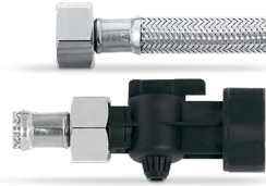
Manguera de admisión DN 13 3/4" - 1" válvula de cierre
